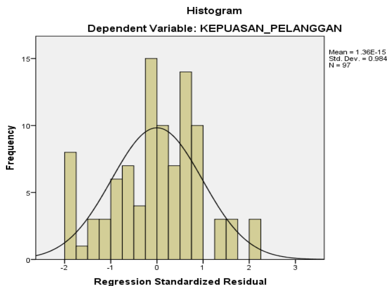
Gambar 1. Hasil UjiNormalitas
